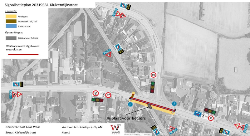
Signalisatieplan fase 1 (klik op de afbeelding voor detail)
