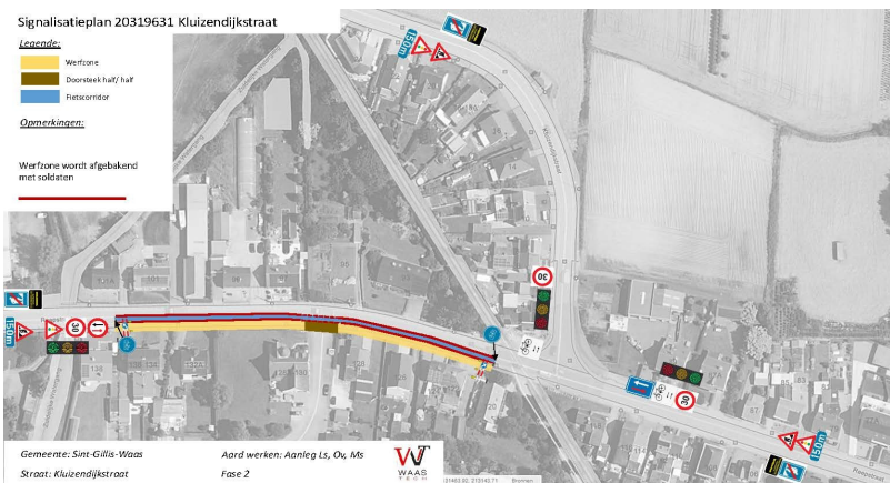
Signalisatieplan fase 2 (klik op de afbeelding voor detail)
