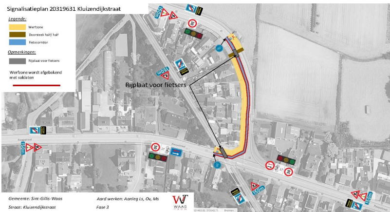
Signalisatieplan fase 3 (klik op de afbeelding voor detail)
